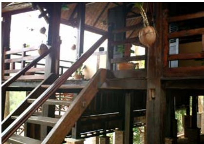
ການໃຊ້ໄມ້ກົມ ແລະ ໄມ້ລຸ່ມເພື່ອເຮັດໂຄງສ້າງເຮືອນພັກ
